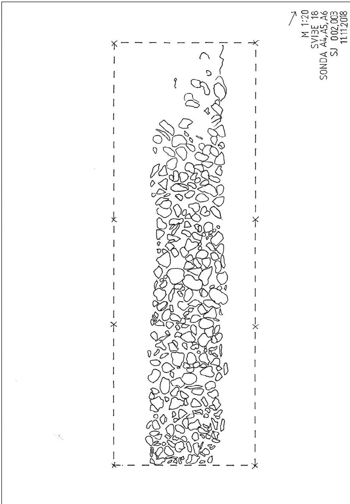
Crtež zidne konstrukcije u sondama A4, A5 i A6 (Crtač: dipl. arh. Amila Očuz)
