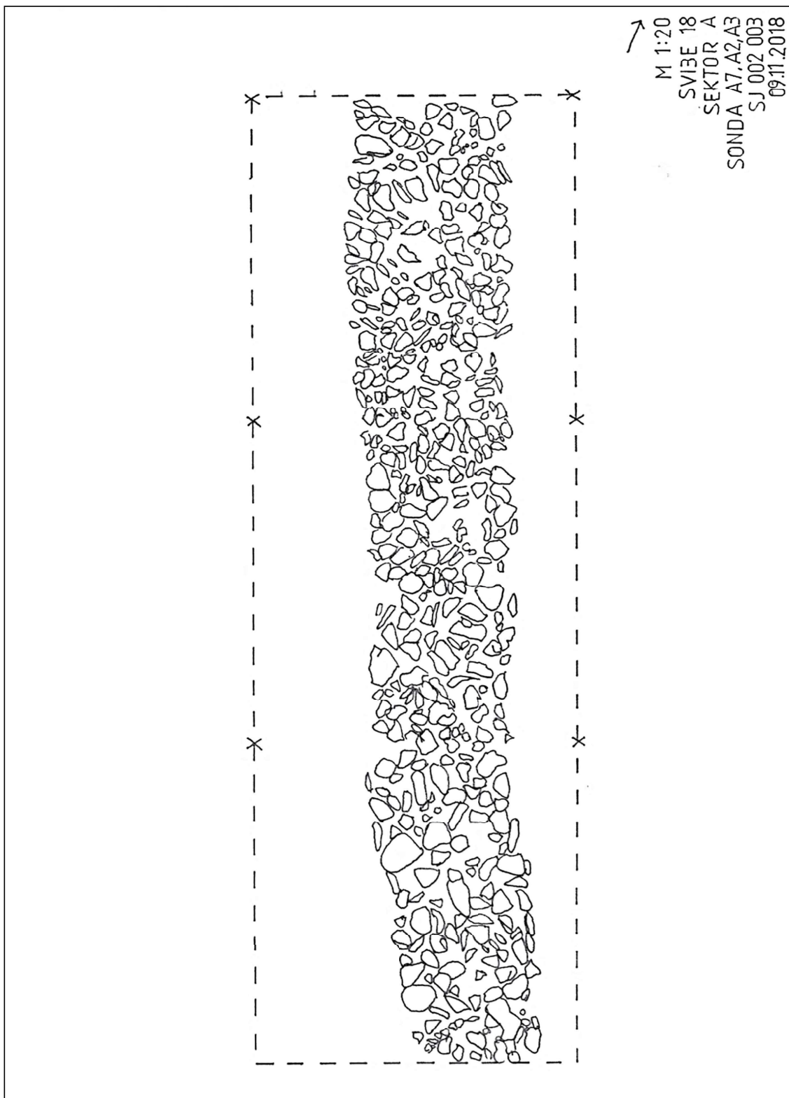
Crtež zidne konstrukcije u sondama A2, A3 i A7 (Crtač: dipl. arh. Amila Očuz)
